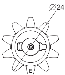
Z=10 m=2
