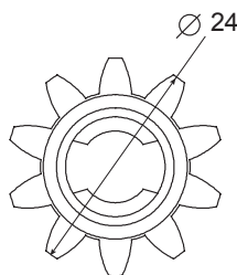
Z=10 m=2
