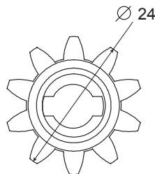
Z=10 m=2
