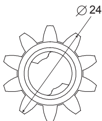
Z=10 m=2
